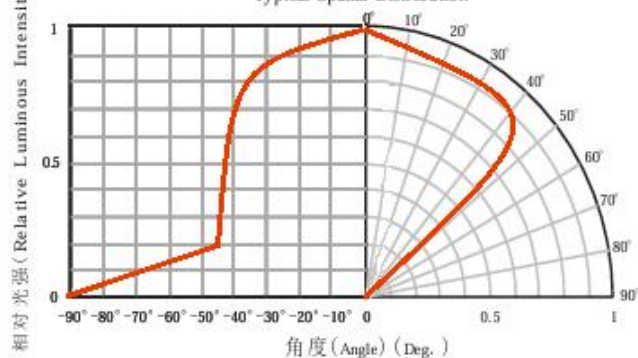
光强分布特性曲线 Typical Spatial Distribution
