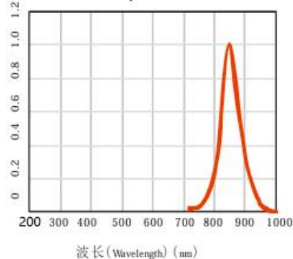
光谱分布特性曲线 Relative Spectral Distribution
