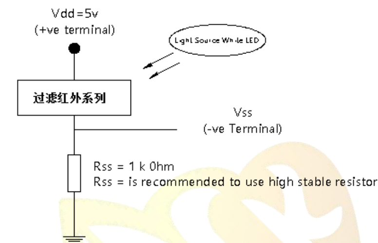
LED通用驱动电路
