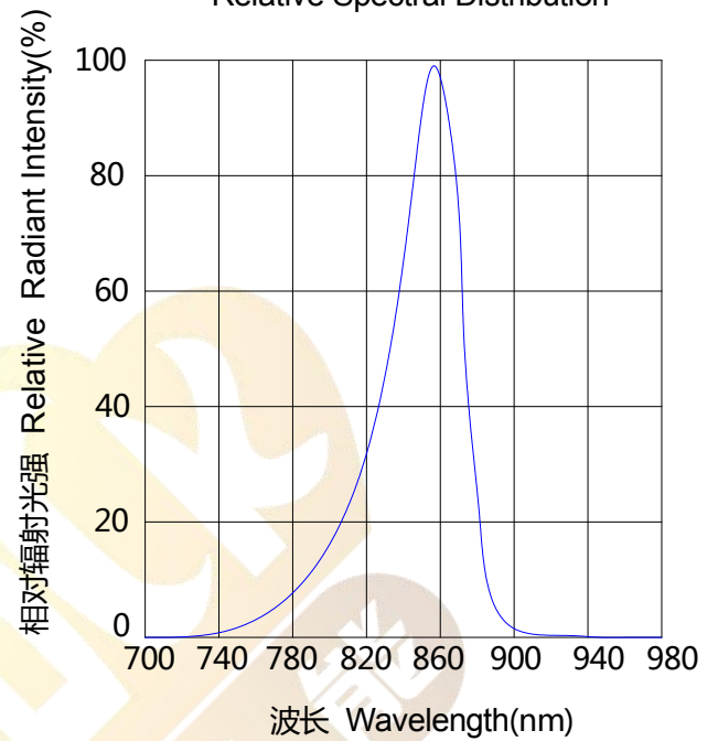
光谱分布特性曲线 Relative Spectral Distribution
