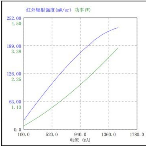
正向电流所对应辐射强度
