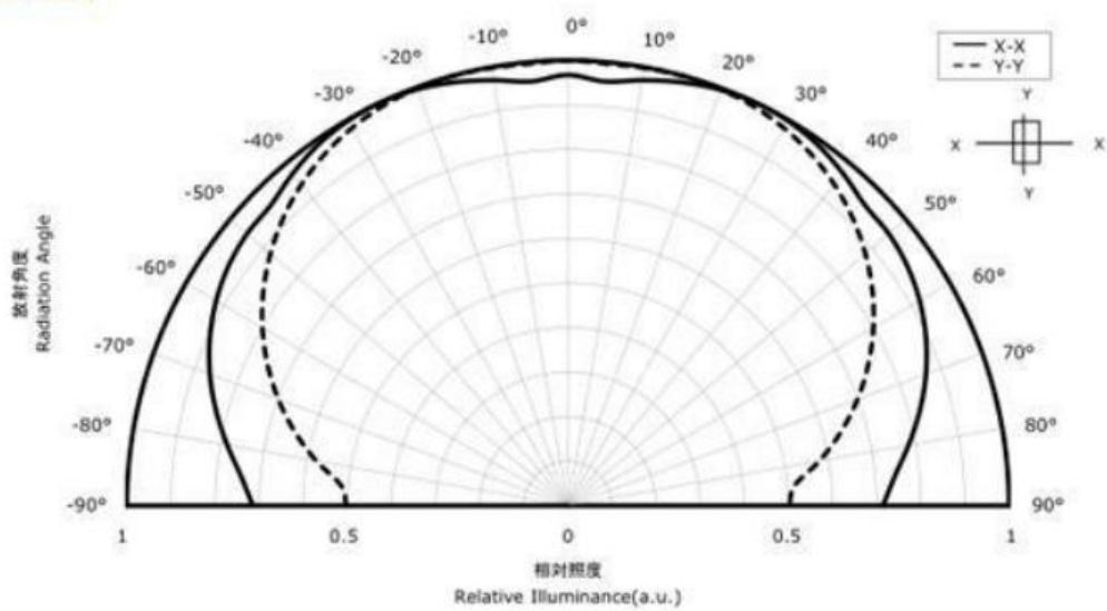
指向特性 Directivity
